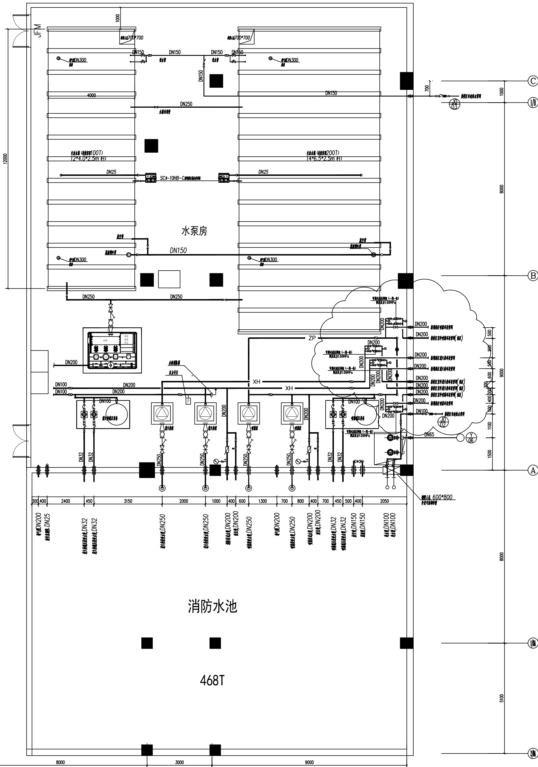
消防、生活水泵房平面大样图 (一) 1:50
